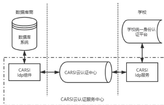
图 1 CARSI 认证原理
