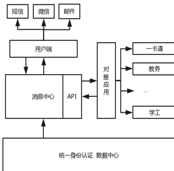
图 1 消息中心架构
