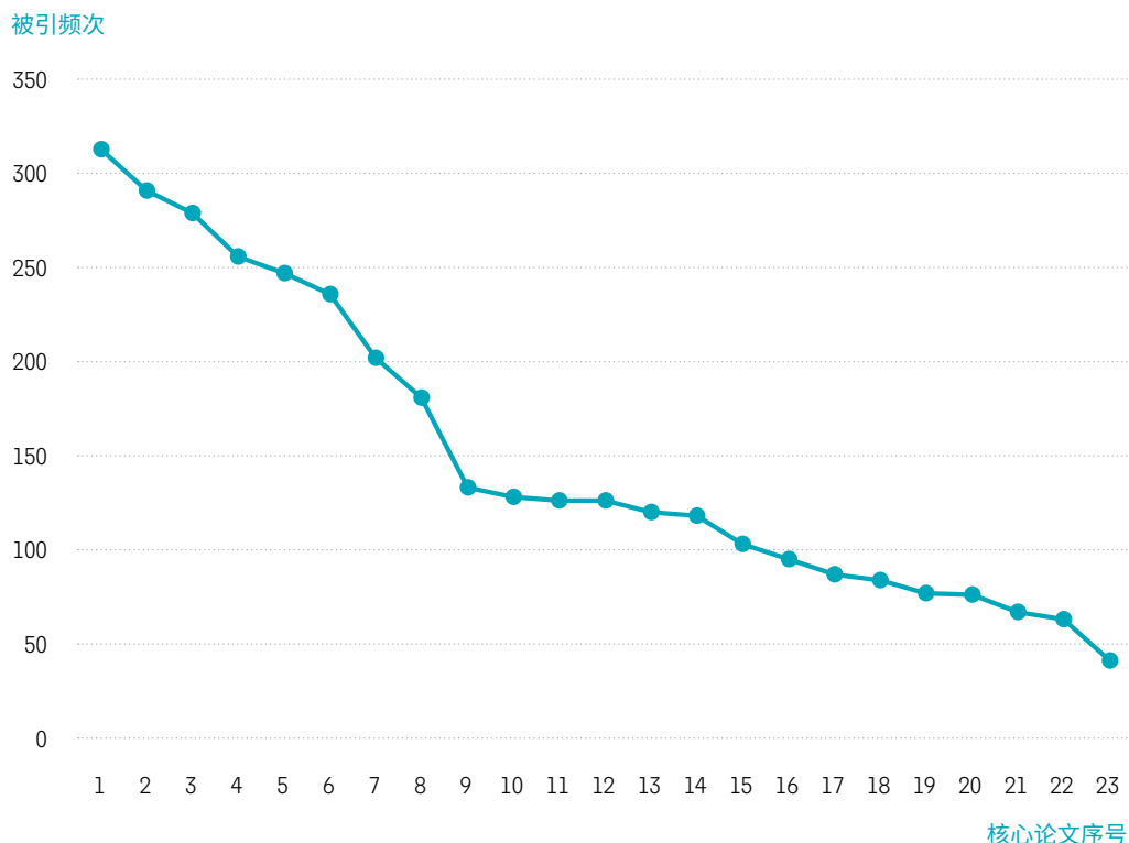
图 17 “磁性拓扑绝缘体 \text{MnBi}_2\text{Te}_4 ” 研究前沿中核心论文的被引频次分布曲线
