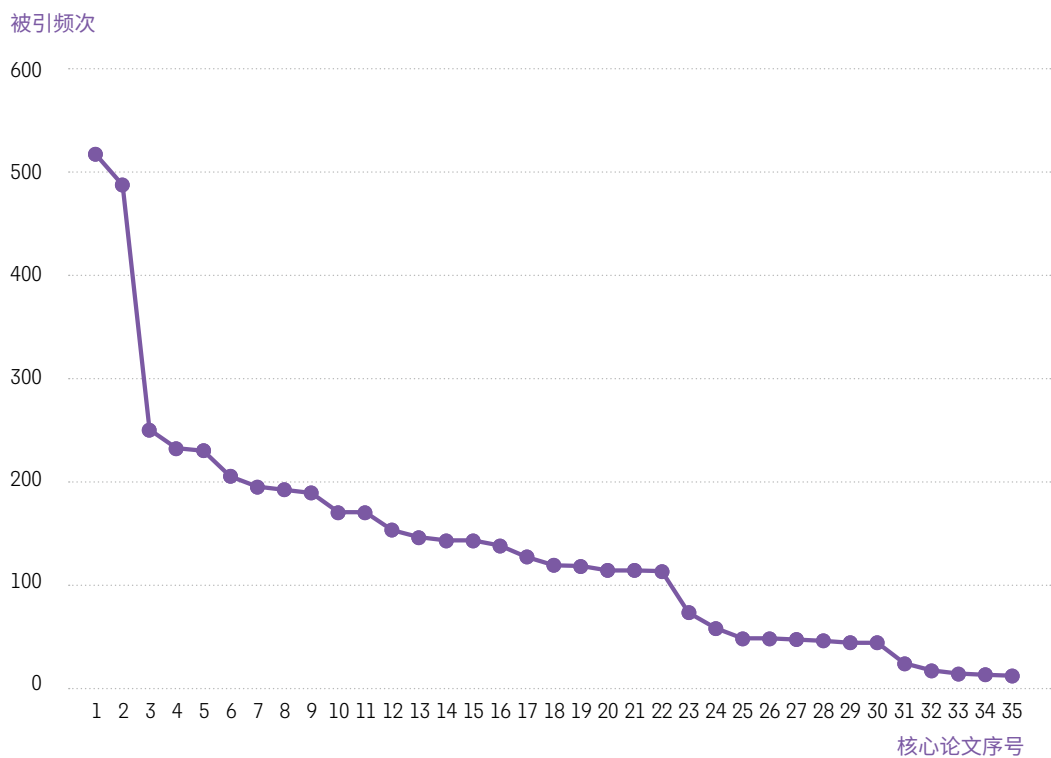
图 15 “机器学习辅助的化学合成”研究前沿中核心论文的被引频次分布曲线
